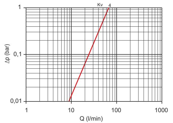
Diagramma portata/perdita di carico Flow/pressure drop diagram
